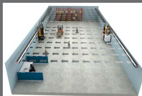
Parallel push-pull systeem met 2 filterunits en 2 ventilatoren
